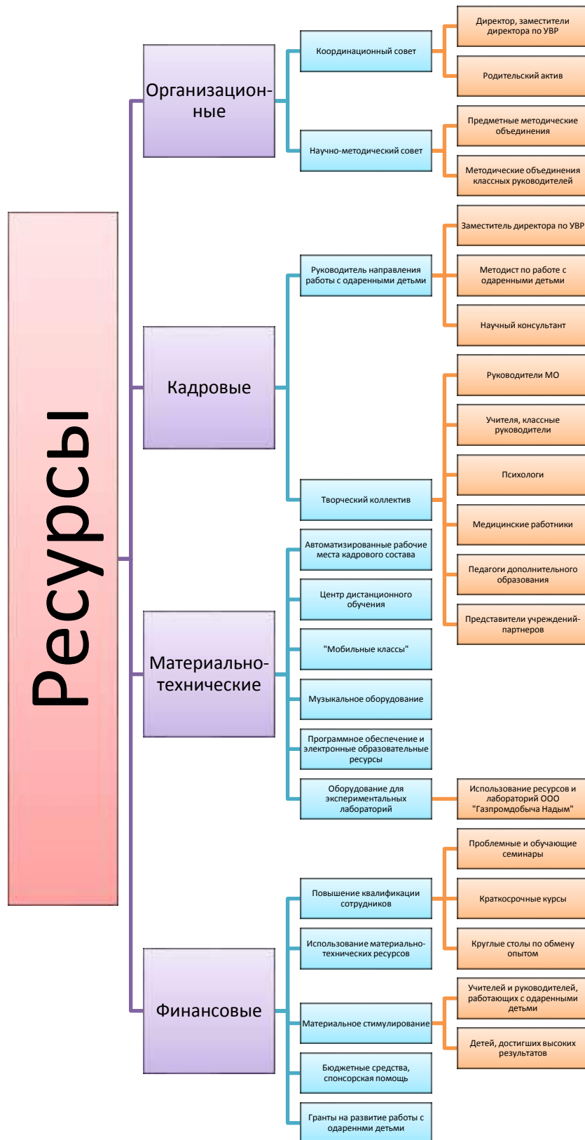
Рисунок 2. Ресурсы программы
